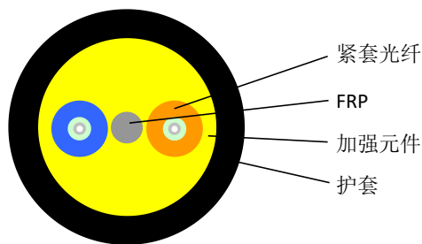
双芯圆形基站光缆 V 型
